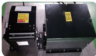
로프브레이크 M100L70
