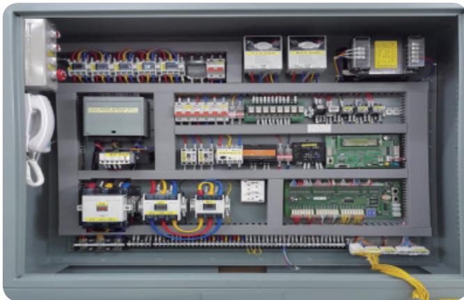
유압식 제어반(ELS-3000F-H)
